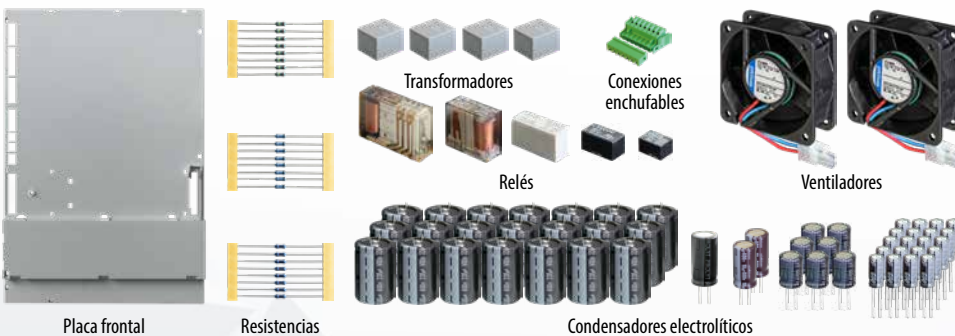
Ejemplo de paquete de reacondicionamiento preventivo para Simodrive 6SN1145*/6SN1146*.
